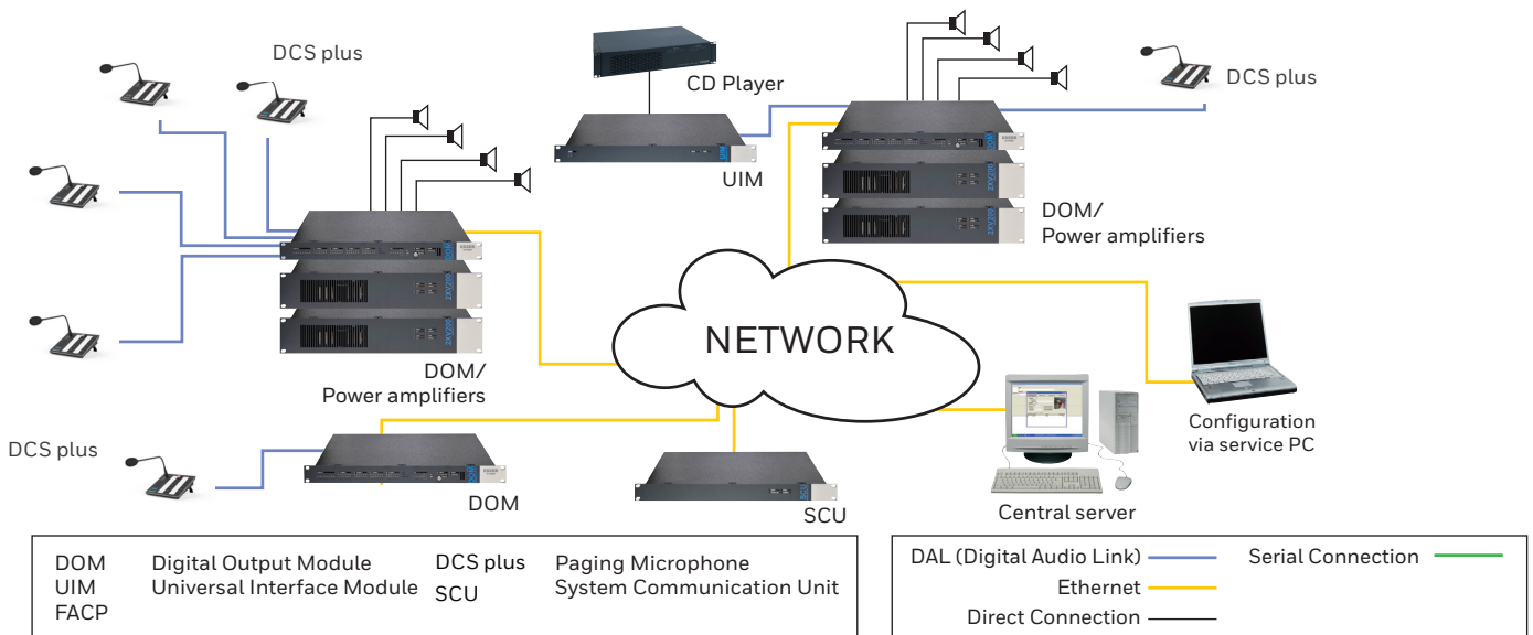
System Overview VARIODYN® D1
